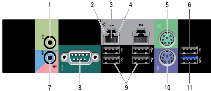
איור 4. תצוגת לוח אחורי
