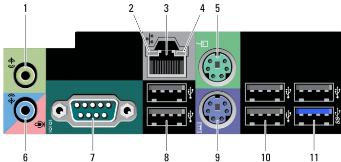
איור 2. תצוגת לוח אחורי
